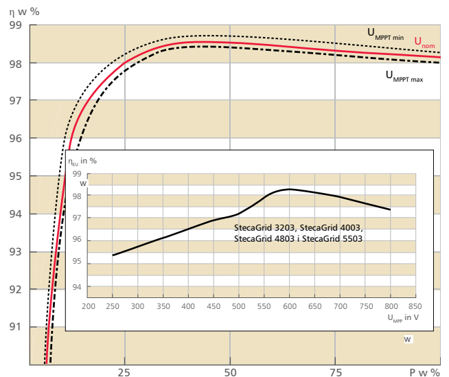
Stożek wydajności falownika StecaGrid 4803 oraz porównanie napięcia MPPT we wszystkich typach
