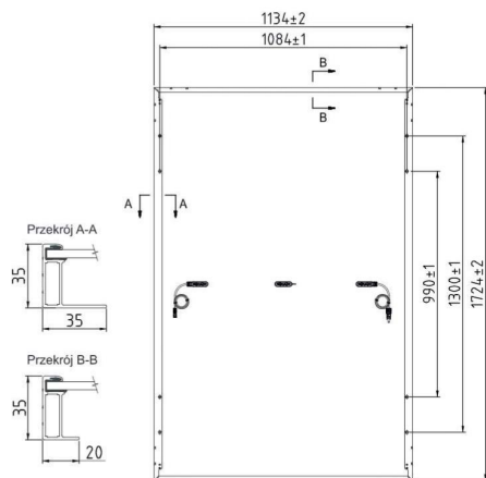
WYMIARY MODUŁU
