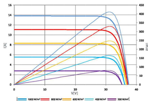
CHARAKTERYSTYKA PRĄDOWO-NAPIĘCIOWA
